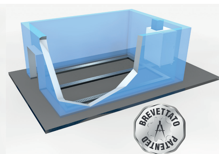
CANALIZZAZIONE A PAVIMENTO ASPIRAZIONE ARIA / SCARICO ACQUA
