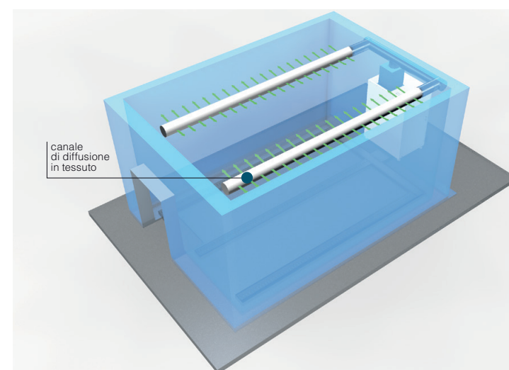
CANALIZZAZIONE AEREA IMMISSIONE ARIA / STAGIONATURA - ASCIUGATURA
